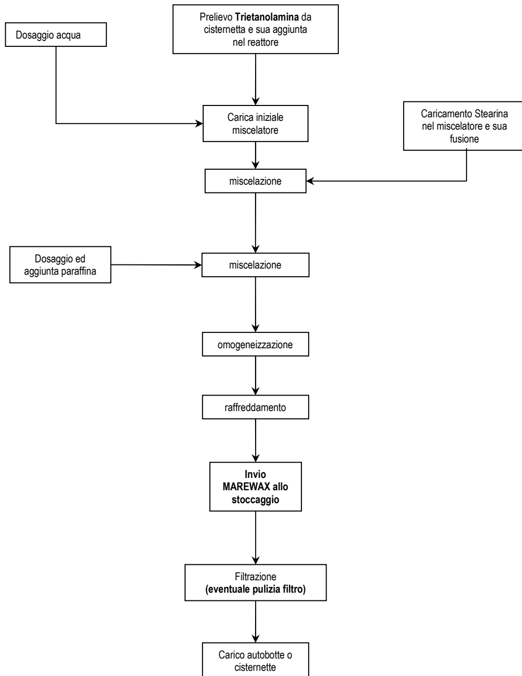
Schema del processo produttivo “Marewax”
