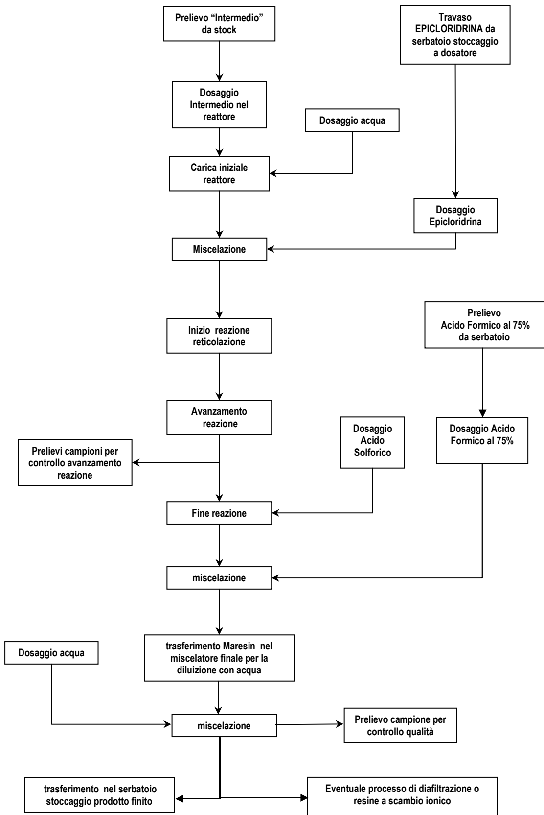
Schema del processo produttivo MARESIN 2
